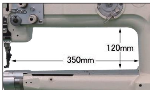
寬闊的工作空間
