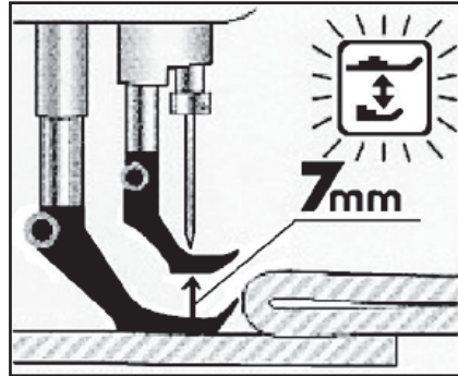
段差部分的平滑縫合 (CD設備)
